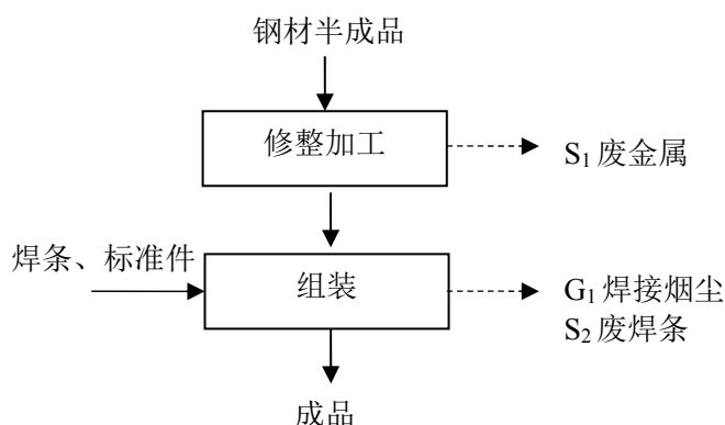
图 2-2 通用机械生产工艺流程图
